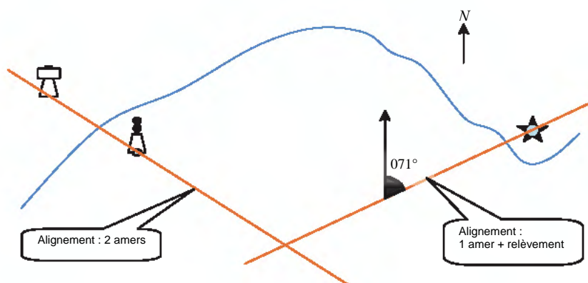
Fig. 23 : Positionnement à l'aide d'amers
