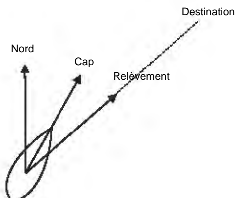
Fig. 17 : Comparaison cap/relèvement
